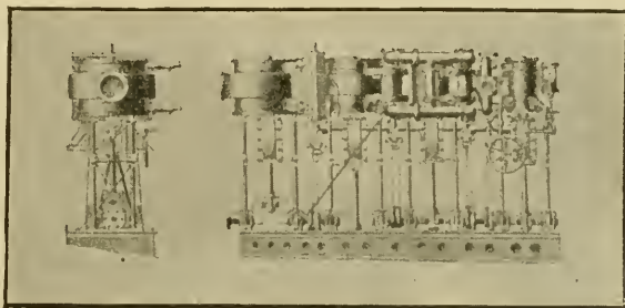
PLATE IV. ENGINE OF U. S. S. ERICSSON.
